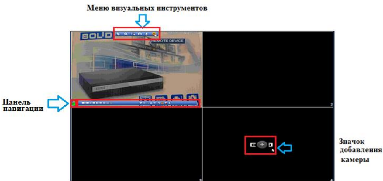
Рисунок 7.3 Добавление IP-камер.
