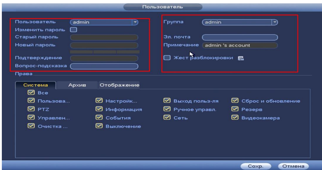
Рисунок 8.114 Добавление пользователя.
