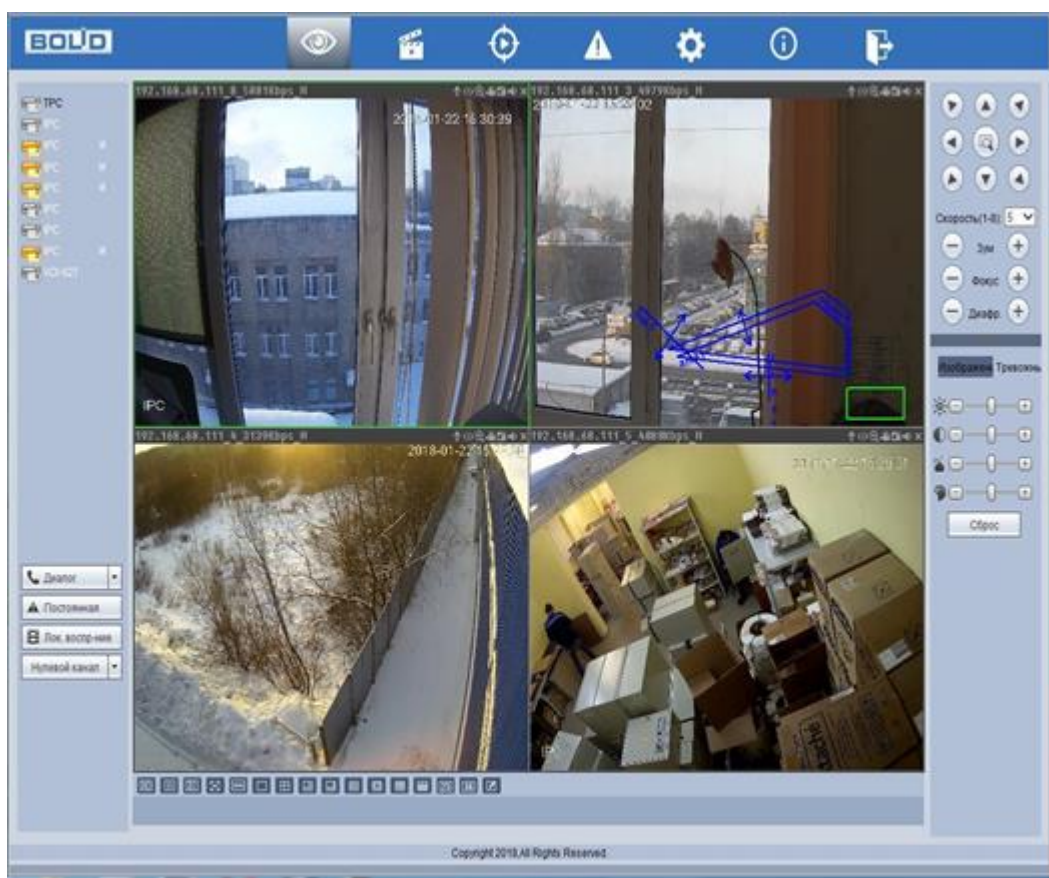
Рисунок 2.1 Web-интерфейс
