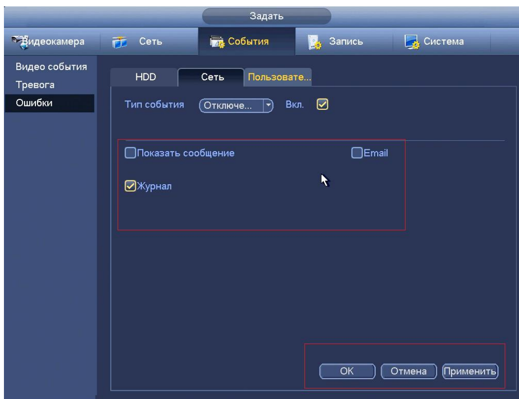
Рисунок 8.87 Установка настроек.
