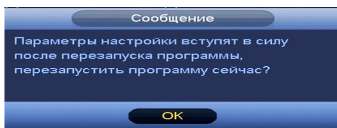
Рисунок 8.100 Всплывающее сообщение.
