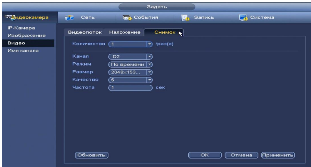
Рисунок 8.40 Настройка снимка.
