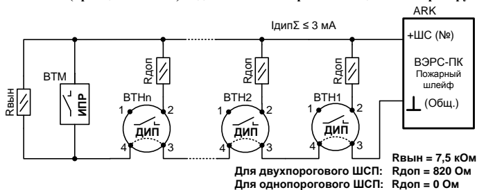
Рисунок.Б3. Схема ШСП типа ШННС и ШПНС с несколькими дымовыми извещателями ВТН (типа ИП212).
